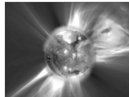
Корональный выброс на Солнце
