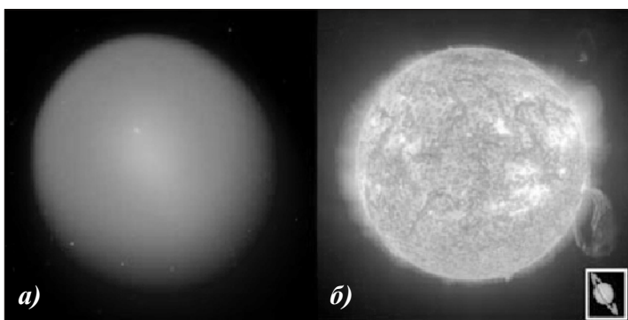
Сравнительные размеры: а) комета Холмса и б) Солнце
