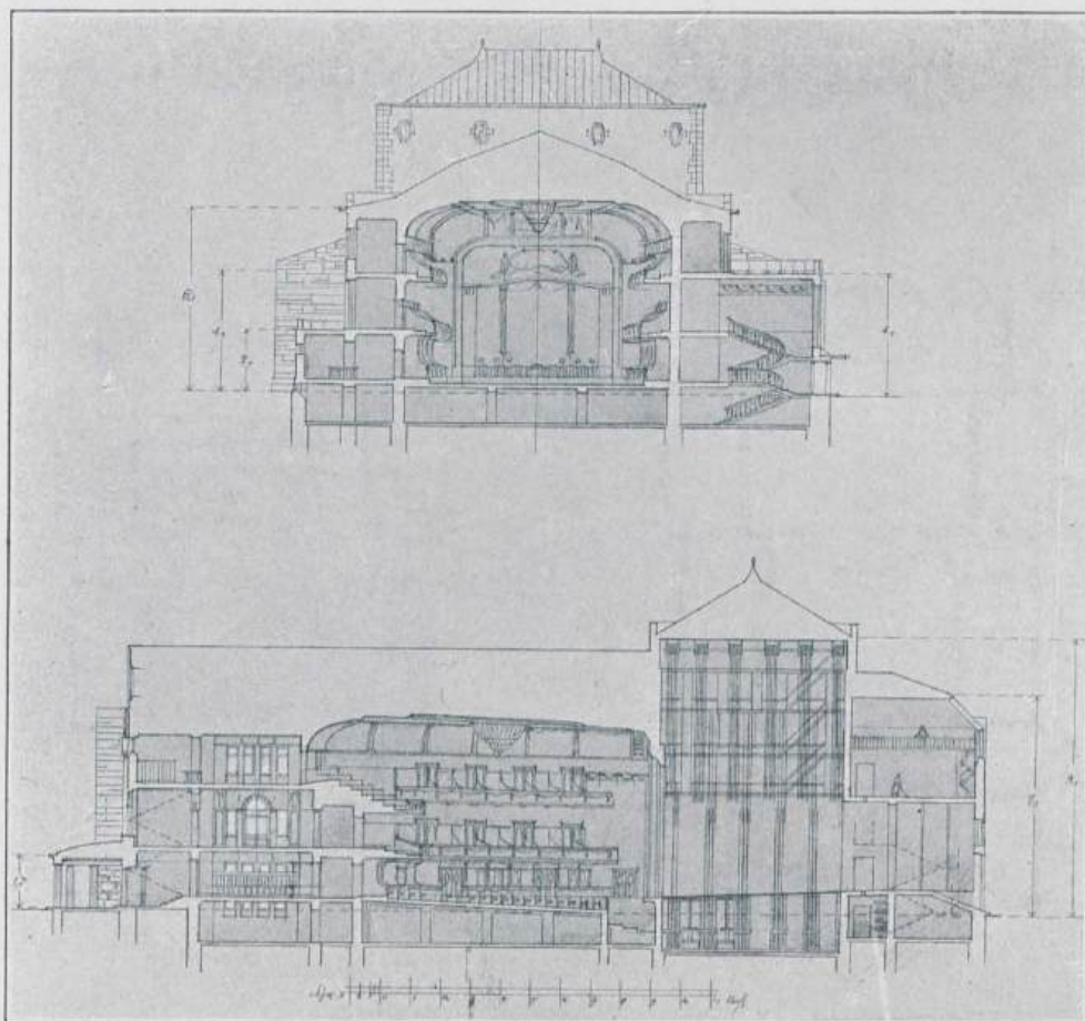
Проектъ театра на 1000 человекъ. Боковой фасадъ и разръзы. О. Р. МУНЦЪ, Художн.-Архитект. и С. В. БЪЛЯЕВЪ, Художн.-Архитект. С.П.Бургъ.
