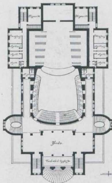
Планъ сцѣны и зрительнаго зала.
