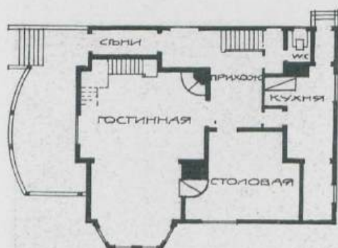
ПЛАНЫ 1-го эт.
