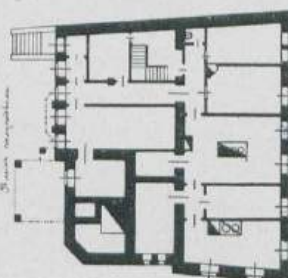
С. У. СОЛОВЬЕВЪ, Домъ-особнякъ. Рыбевскій пер., Москва. Деталь входа и планы. А. А. АНДРЕЕВЪ, Художн. скульпт. Москва.
