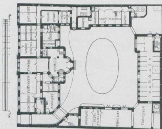
ПЛАНЫ 1-го ЭТАЖА
