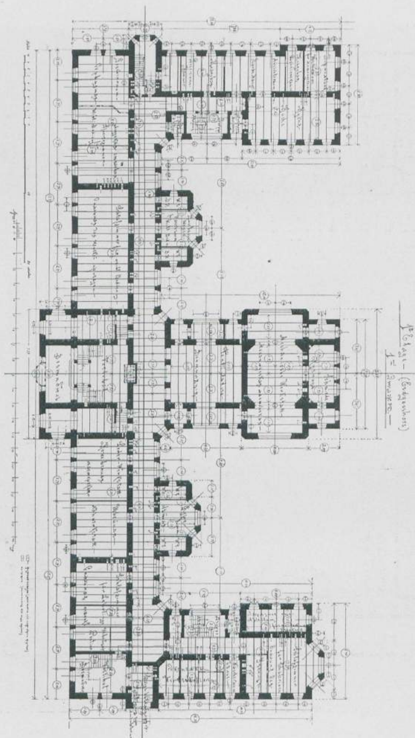
С.-Петербургскій Ортопедическій Институтъ. Александровскій паркъ. С.-Петербургъ. Планъ 1-го этажа. Р. Ф. МЕЛЬЦЕРЪ, Художн.-Архитектъ. С. П. ВѢРГЪ.
