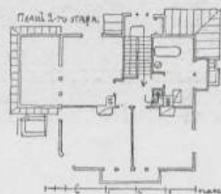
Дача въ поселкѣ Ольгино. Ключевой пр., Лахта, С.-Петербургъ. А. П. ВАЙТЕНСЪ, Художл.-Архитект. С.П.Бургъ.
