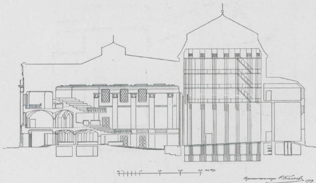
Проектъ народнаго театра для г. Риги на 1800 чел. (2-я премія на международномъ конкурсѣ). Главный фасадъ и продольный разрезъ. С. В. БѢЛЯЕВЪ, Художн.-Архитект. С. П. Бургъ.
