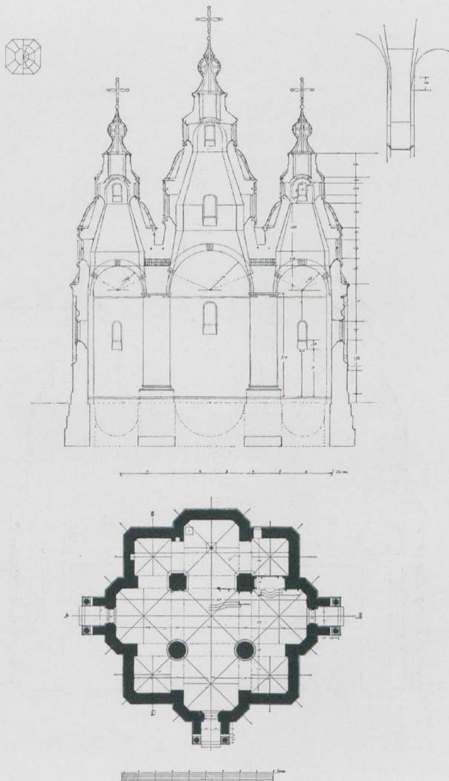
Ц. въ с. Плѣшивцахъ, Полтавской г., Гадячскаго у. Разрѣзъ по боковому наосу и планъ. И. С. КУЗНЕЦОВЪ, Художн.-Архитект. Москва.
