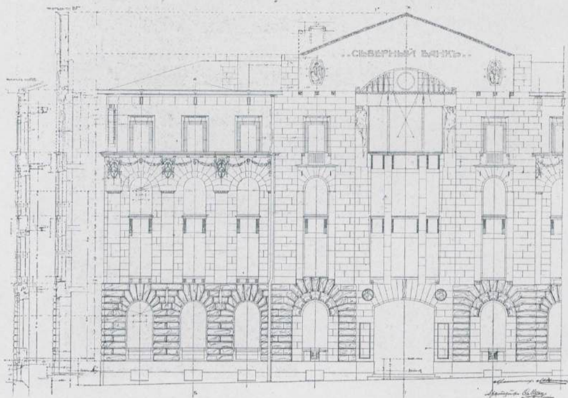
Проектъ здания для Отдѣленія Сибирскаго Банка въ Харьковѣ. Детали фасадовъ. А. К. ШПИГЕЛЬ, Художн.-Архитект. и О. Р. МУНЦЪ, Художн.-Архитект. С.П.Бургъ.
