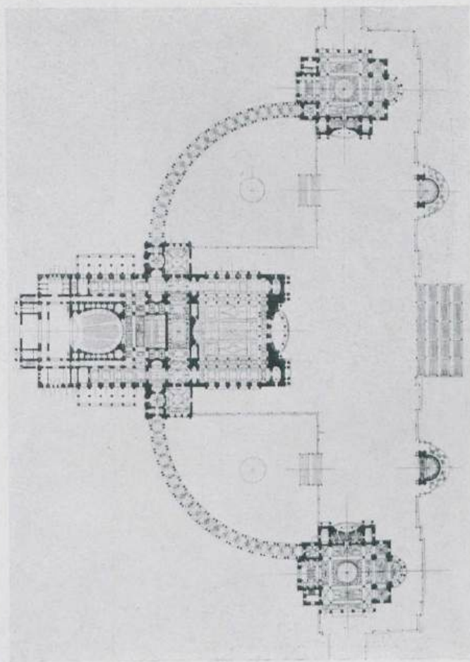
Бирзалъ. Академическая программа 1909 г. (автору присуждена заграничная поездка). И. А. ФОМИНЪ, Художн.-Архитект.
