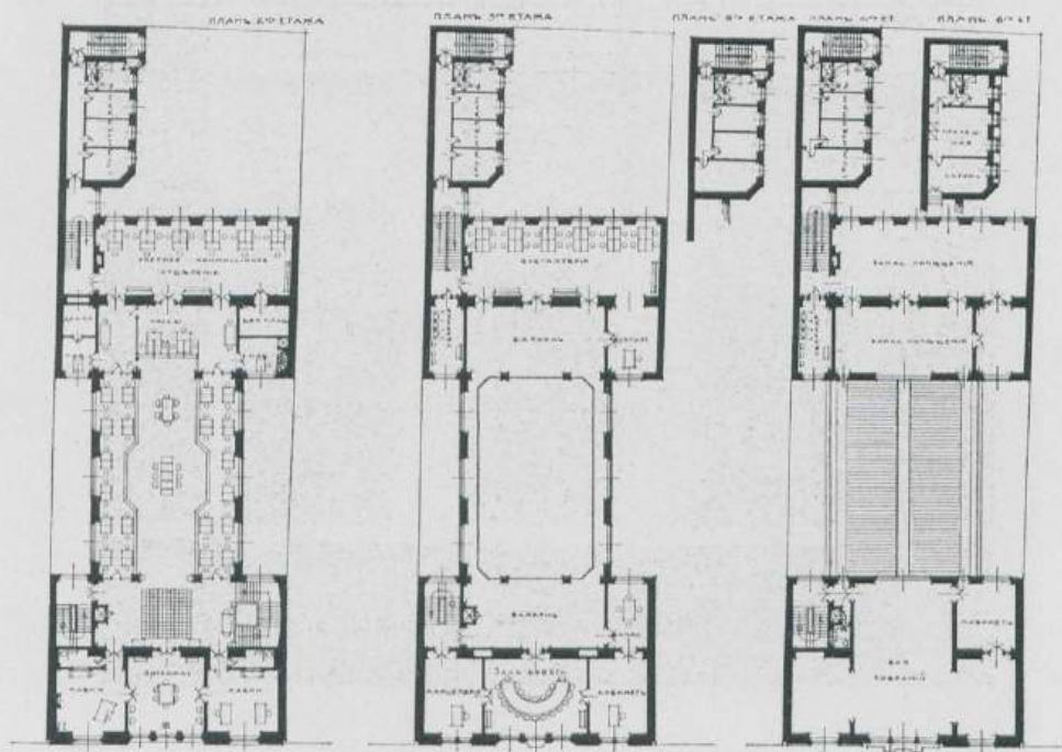
2-е С.-Петербургское Общество Взаимнаго Кредита. Садовая, С.-Петербургъ. Планы. Ф. И. ЛИДВАЛЬ, Академикъ Архитектуры, С.П.Бургъ.
