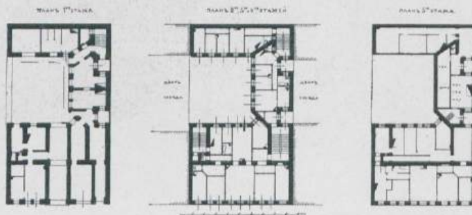
Домъ Н. А. Вязлова, Можайская ул., С.-Петербургъ. Фасадъ и планы. Л. Л. ШРЕТЕРЪ, Художн.-Архитект. С.П.Бургъ.
