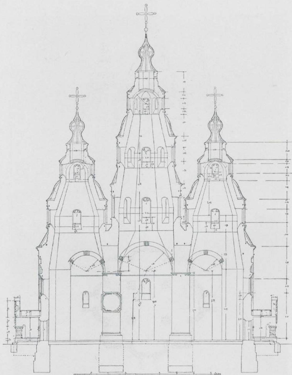
Ц. въ с. Платишцахъ, Полтавской г., Гадячскаго у. Поперечный разрезъ черезъ среднй наосъ. И. С. КУЗНЕЦОВЪ, Художн.-Архитект. Москва.
