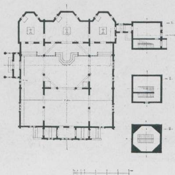
Проектъ деревянной церкви на 750 человекъ въ имѣніи Мансуровыхъ, Тамбовской губ. Разрѣзъ и планъ. А. В. ШУСЕВЪ, Художн.-Архитект. С. П. Бургъ.
