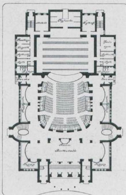
Планъ партера.
