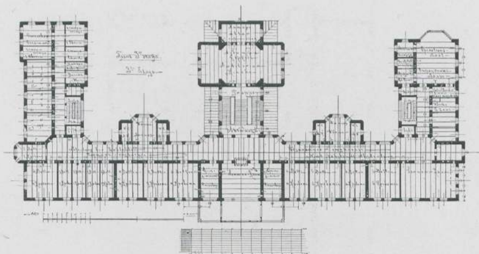
С.-Петербургскій Ортопедическій Клиническій Институтъ. Александровскій паркъ. С.-Петербургъ. Планъ III-го этажа. Р. Ф. МЕЛЬЦЕРЪ, Художн.-Архитект. С.П.Бургъ.
