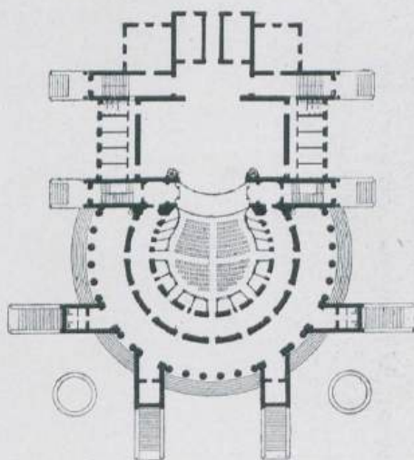
Проектъ театра. Фасадъ, разръзъ и планъ. Академическая отчетная выставка 1909 г. С. С. СЕРАФИМОВЪ.
