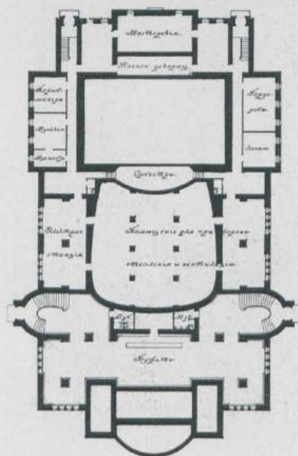
Планъ партера.
