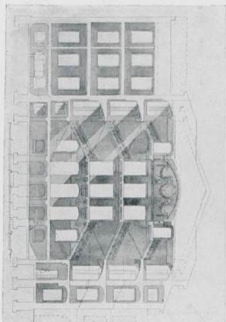
Здания Государственной типографии въ С.-Петербургѣ. Петерб. сторона. Оранienbaumская ул. Генеральный планъ 1-го этажа, часть фасада съ проездомъ и разрывъ. Л. Н. БЕНУА, Профессоръ Архитектуры. С.П.Бургъ.
