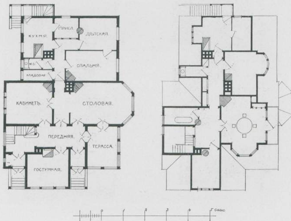
Проектъ дачи на Лахтѣ (близъ С.-Петербурга). Планы. Г. Е. ГИНЦЪ, Художн.-Архитект. С.П.Бургъ.
